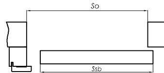
drzwi przesuwne – system naścienny bez zabudowy
